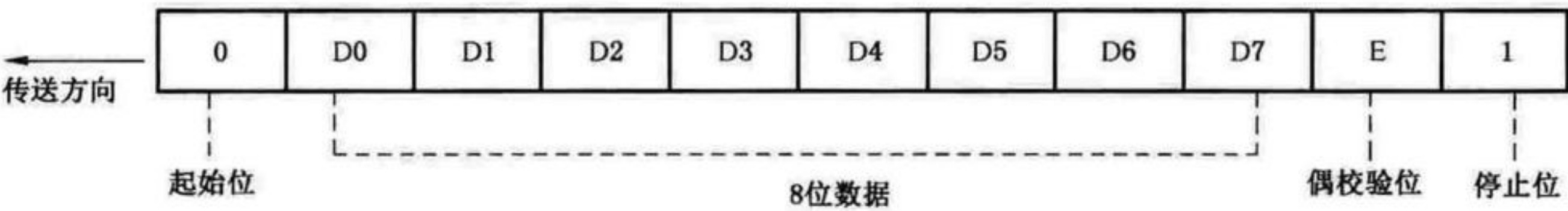
图 2 字节传输序列
