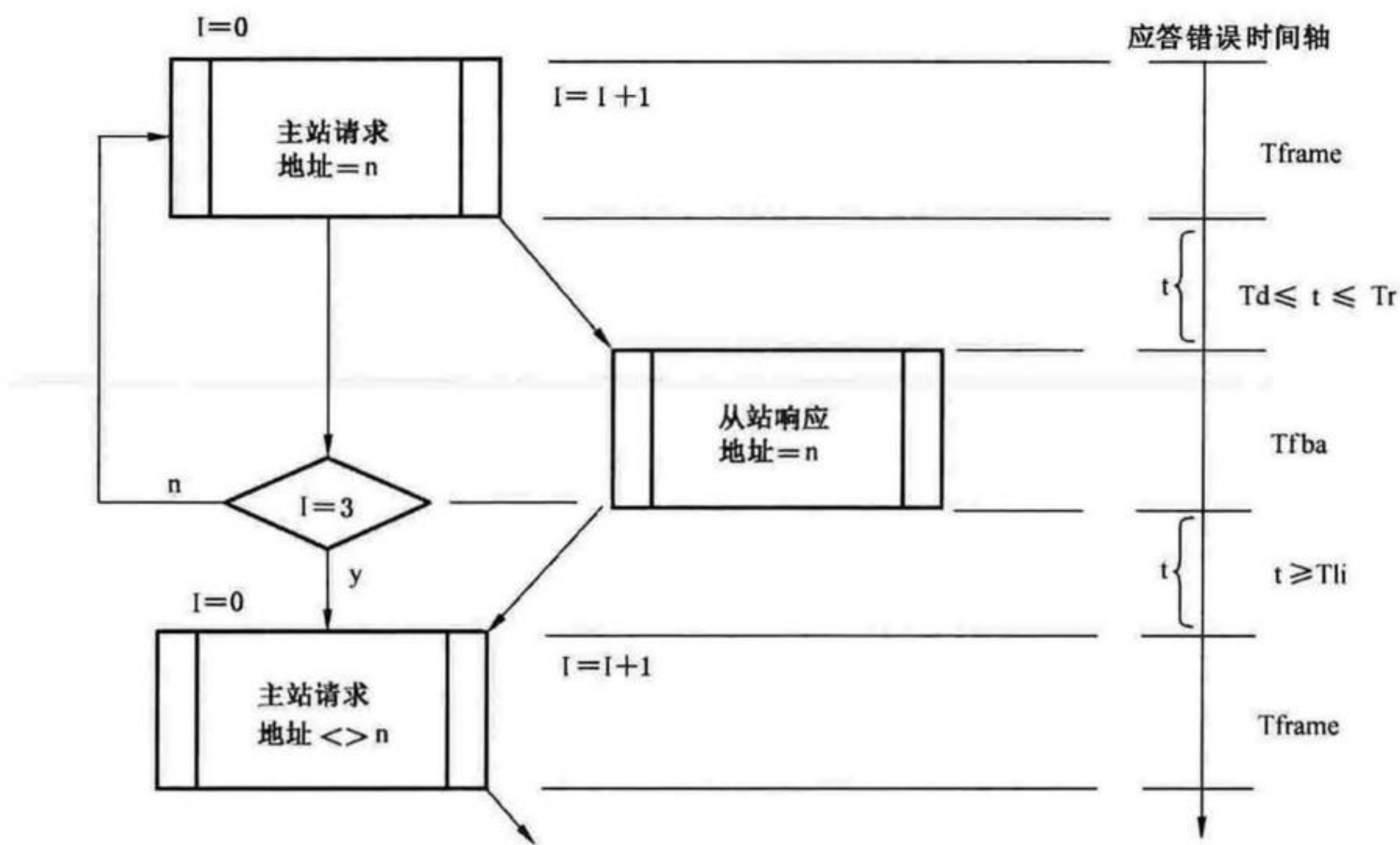
图 6 主站请求应答错误失败时序图
