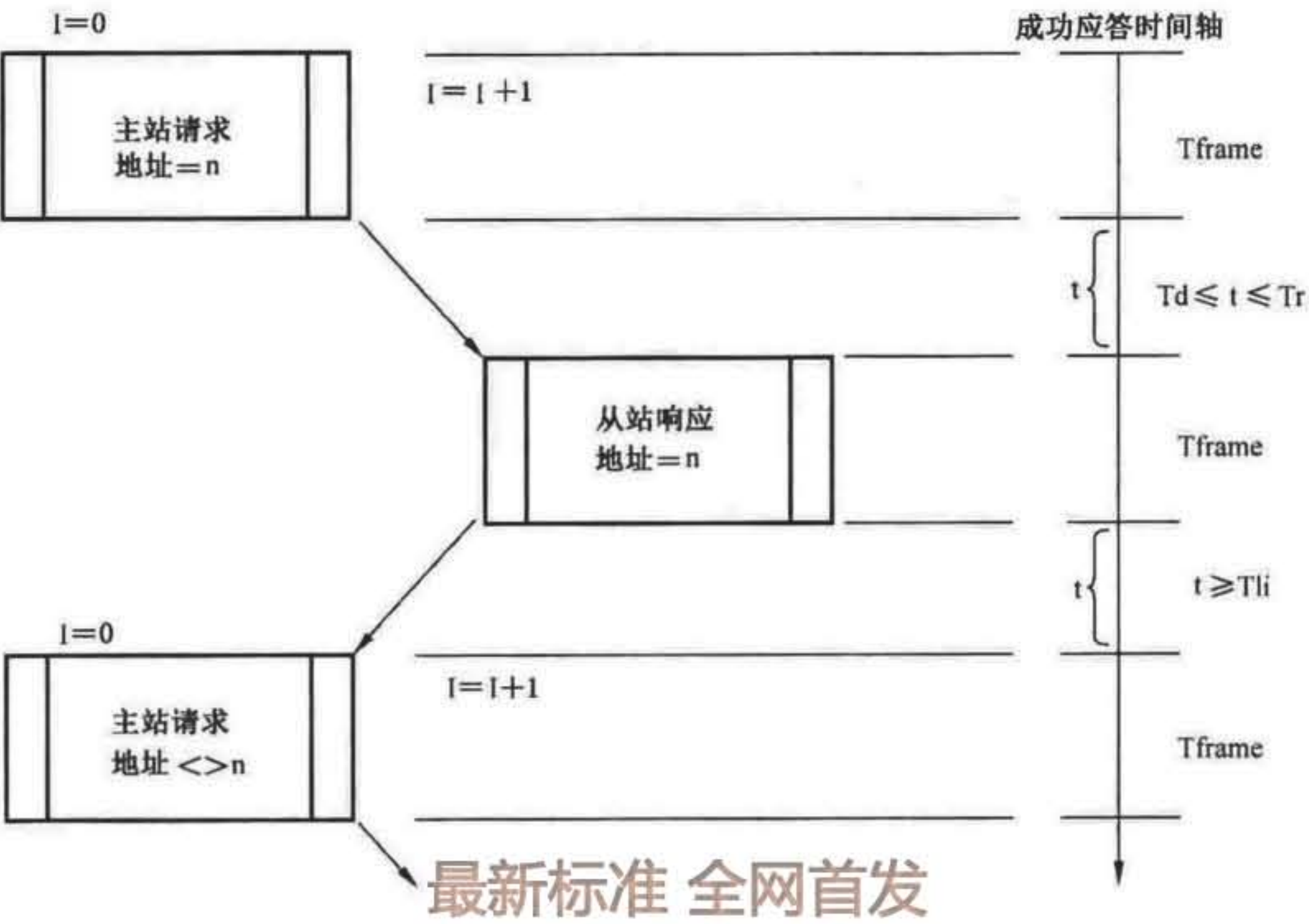
图 4 主站请求成功时序图
